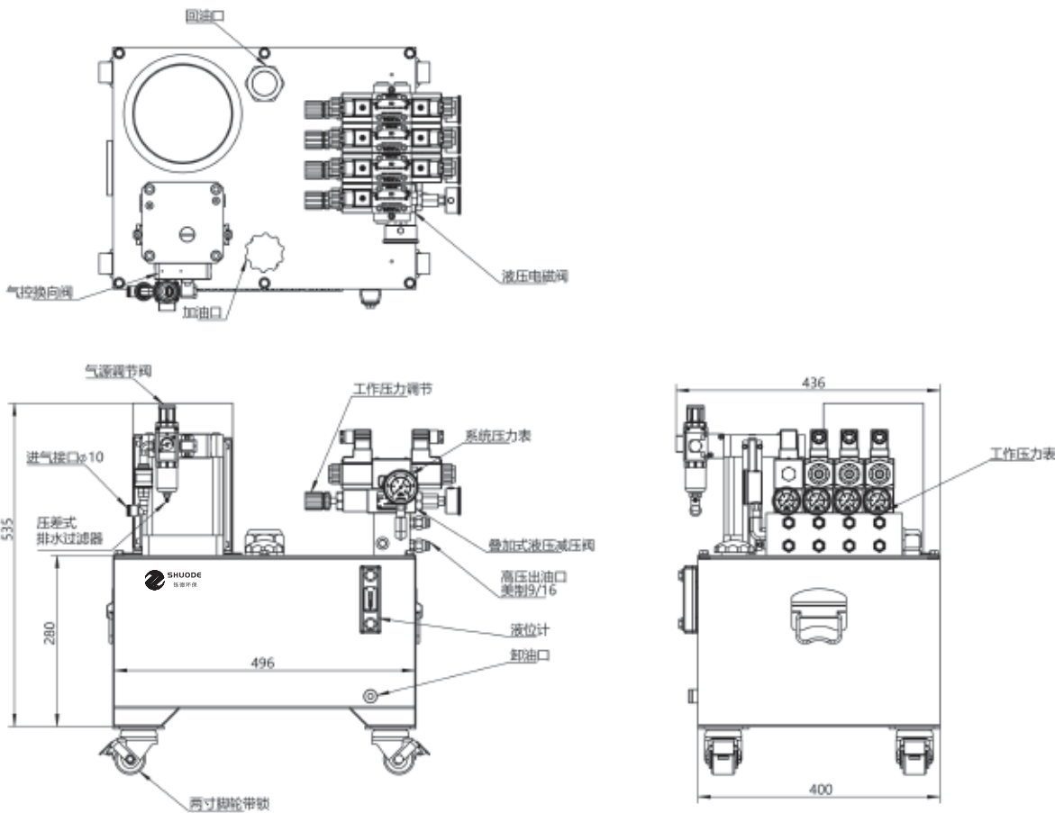
平面结构图 PLANAR STRUCTURE DIAGRAM
