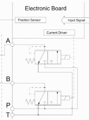
液压原理图
