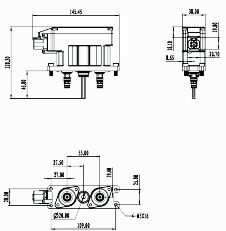
外形图
