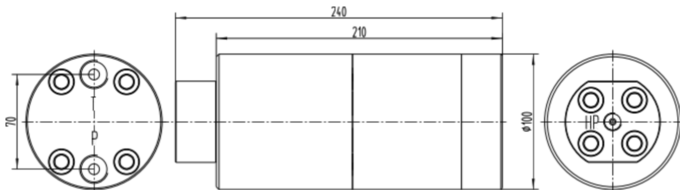
装配示意图
