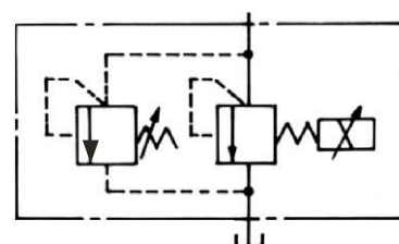
帶安全閥
