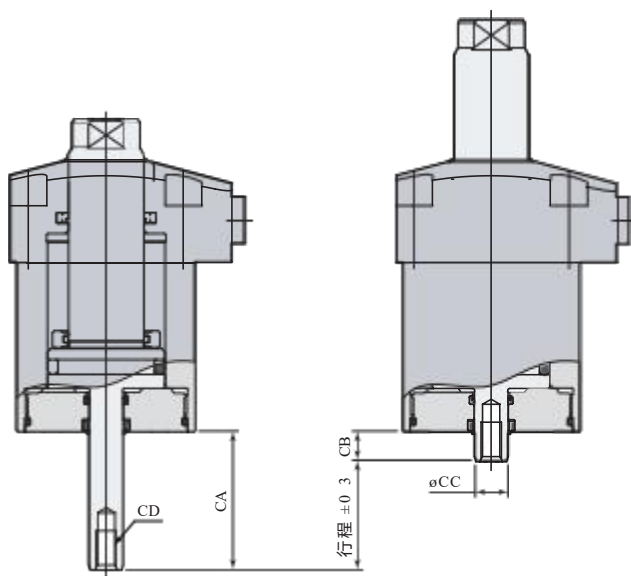
外形尺寸图 双头杆 E 规格
